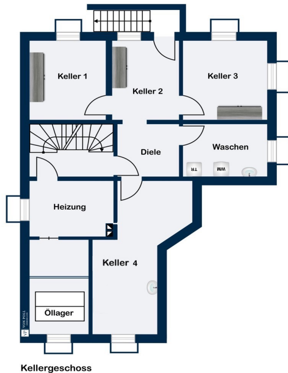
Kellergeschoss
