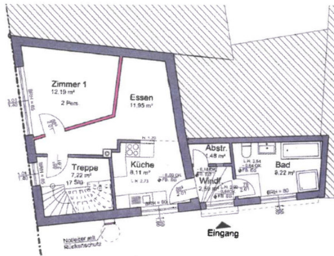
Erdgeschoss (2 Personen)
