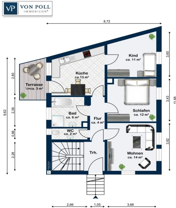
Dachgeschoss
