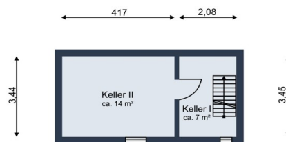
Kellergeschoss
