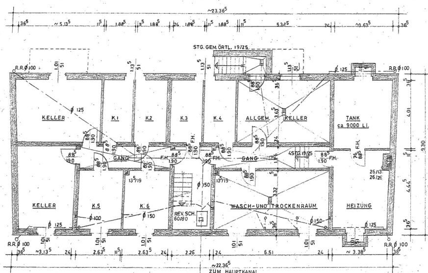
KELLERGESCHOSS M.1:100
