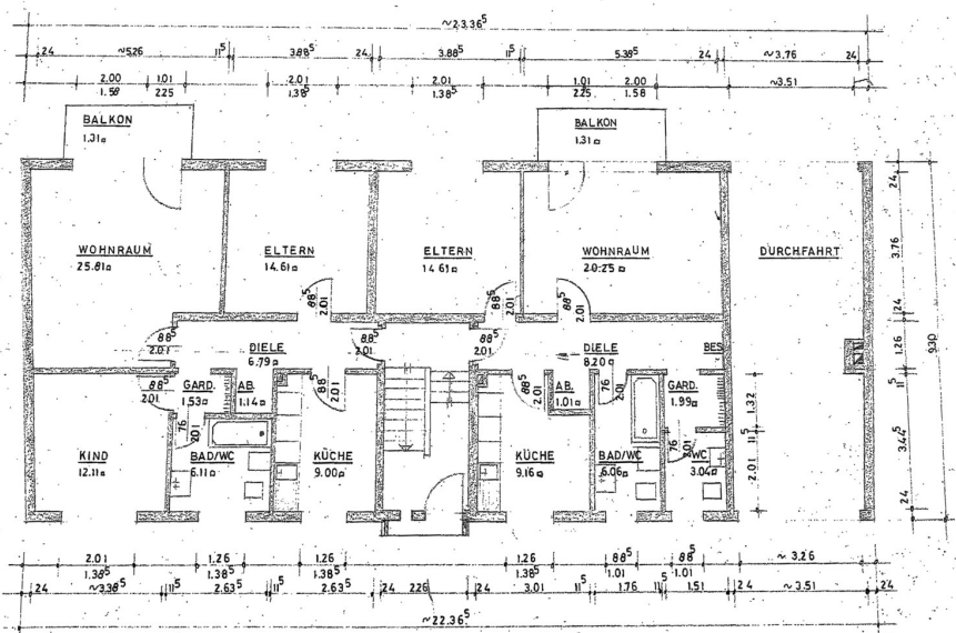
ERDGESCHOSS M.1:100
