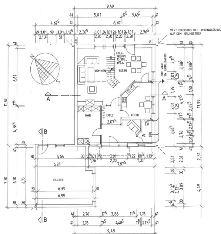
Grundriss Erdgeschoss
