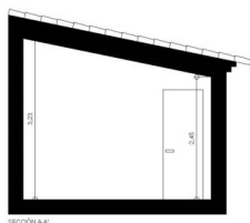
SECCIÓN A-A
