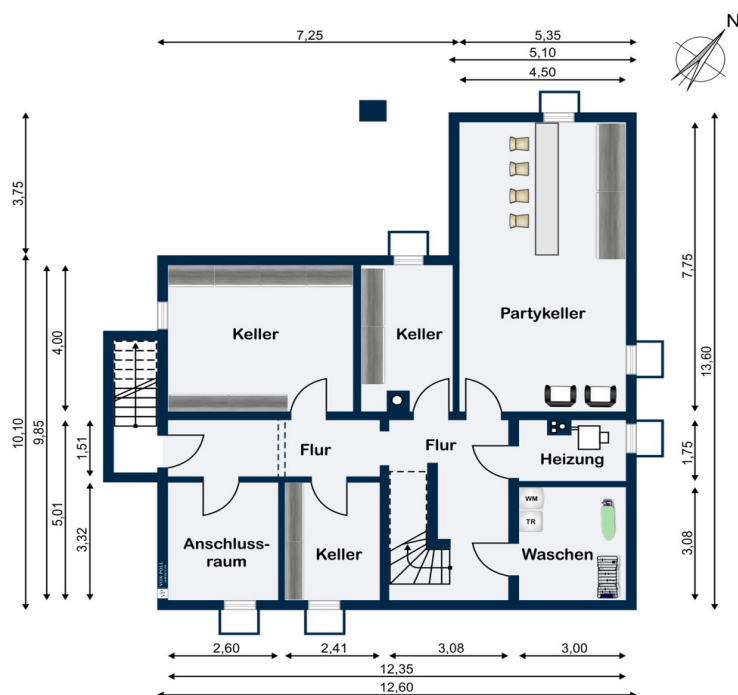
Kellergeschoss
