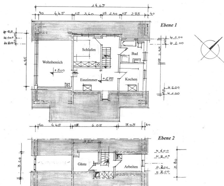
Grundriss Obergeschoss M=1 : 100
