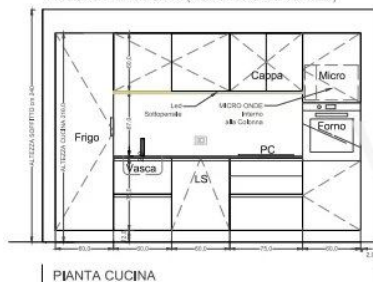
PIANTA CUCINA
