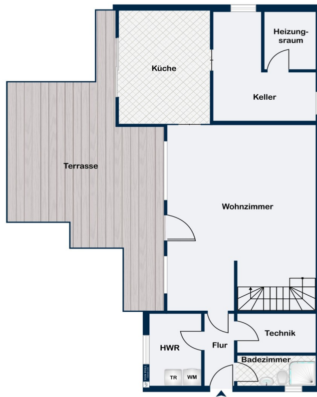
Untergeschoss
