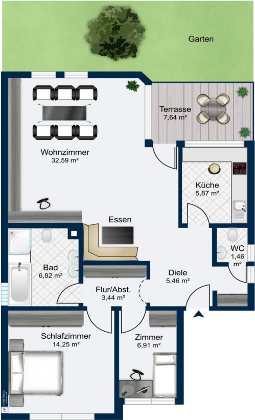
Erdgeschoss
