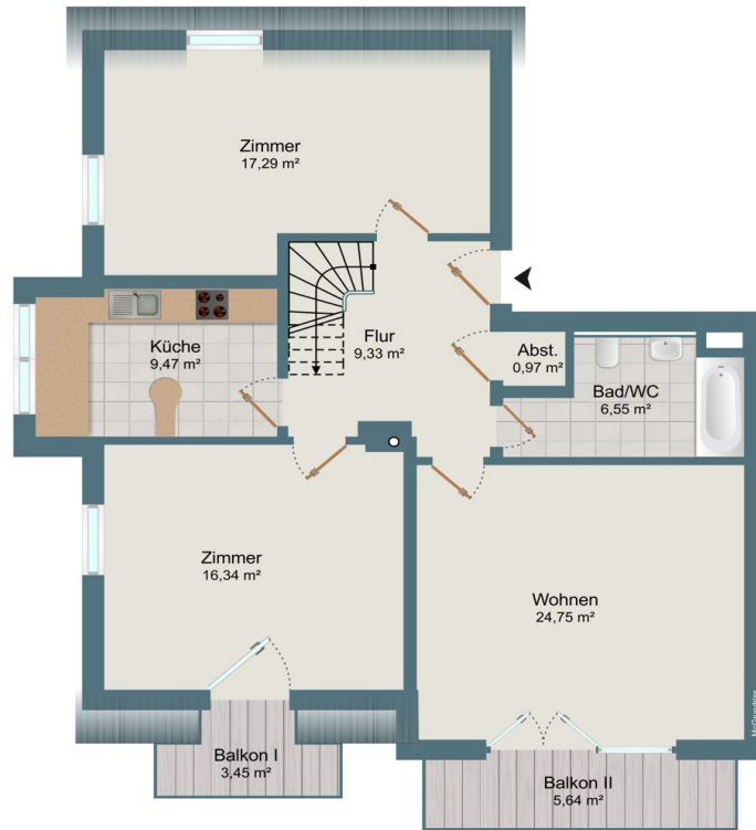
2. Obergeschoss
