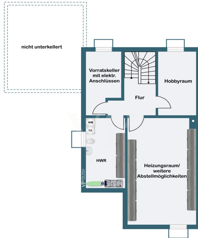
Kellergeschoss
