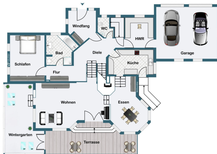
Erdgeschoss
