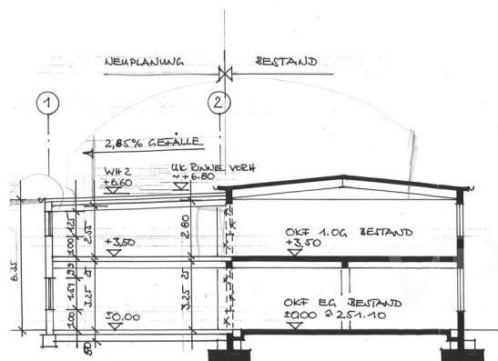
SCHNITT A-A
