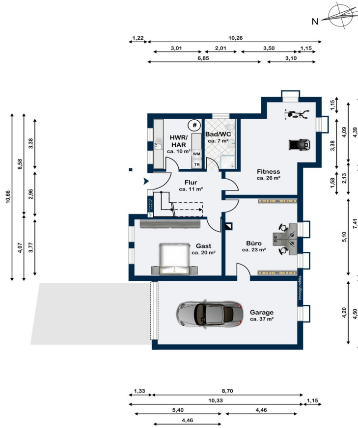
Kellergeschoss
