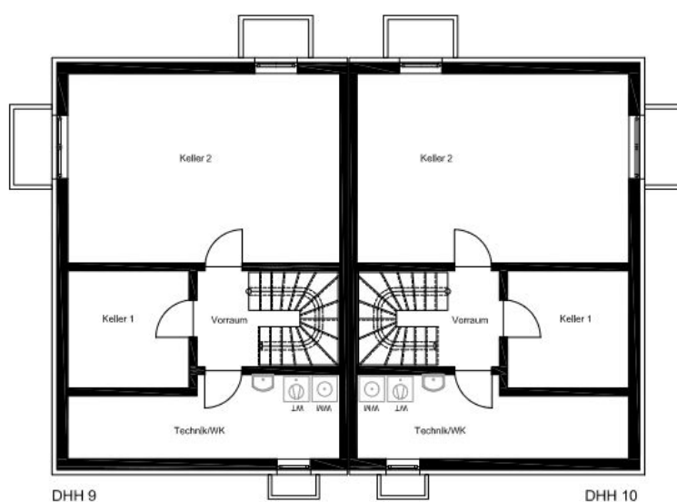
Grundriss UG
