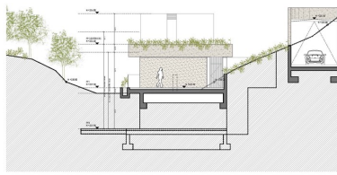
ALZADO 02 - FACHADA NOROCCIDE 1:100
