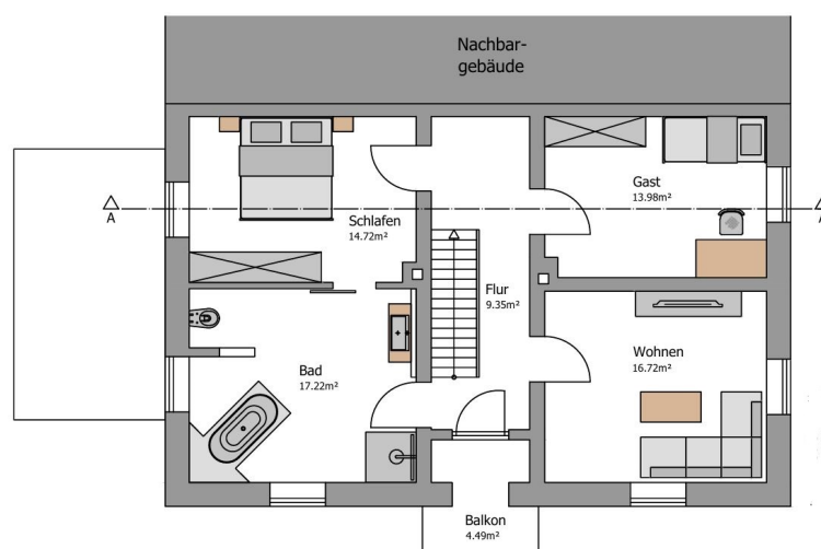
Obergeschoss
