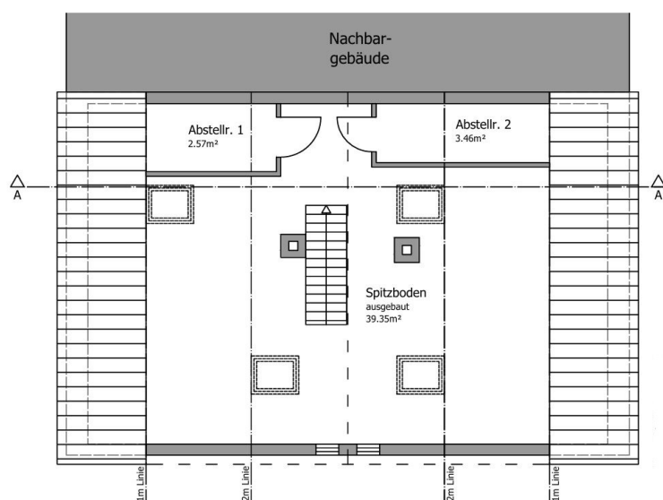
Dachgeschoss
