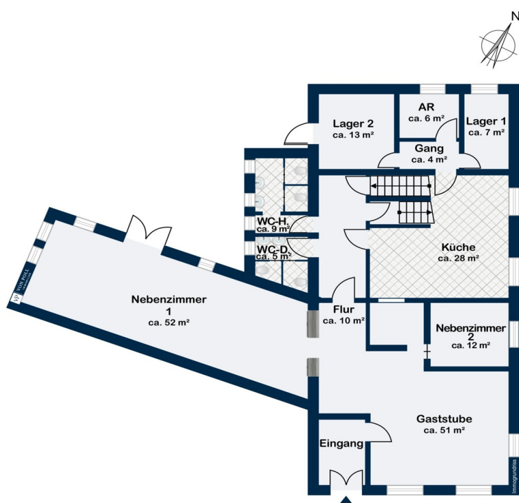
Erdgeschoss
