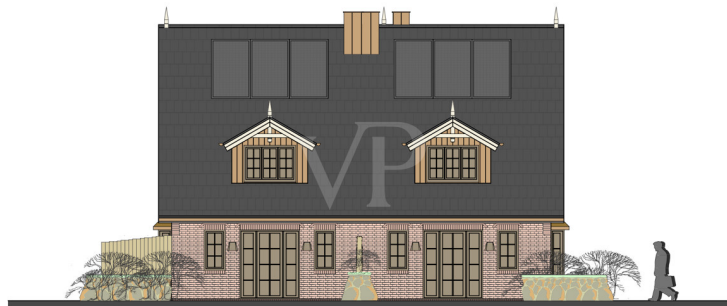
SÜDANSICHT M 1:100
