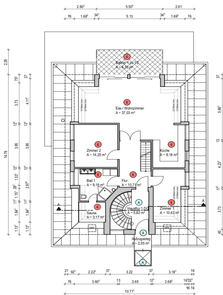
Grundriss 1. Dachgeschoss
