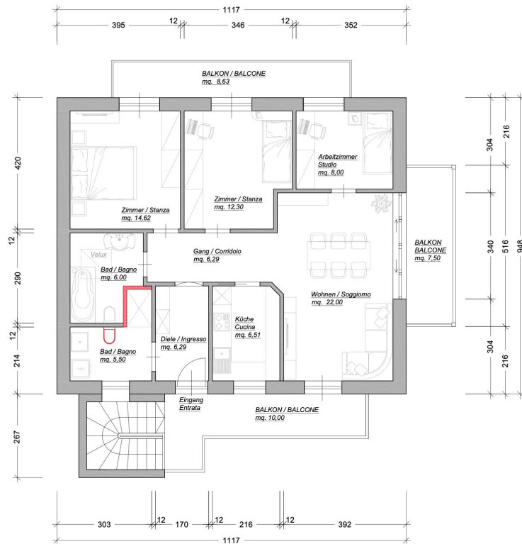
GRUNDRISS / PLANIMETRIA Variante mit zweitem Bad / secondo bagno
