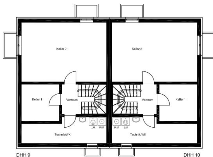
DHH 9 Grundriss UG
