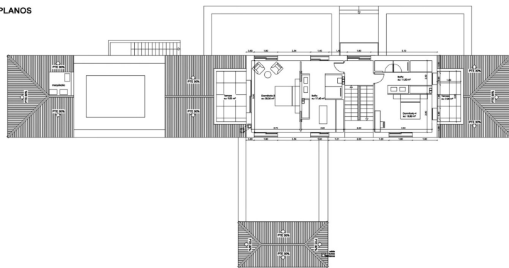
Planta primeira sup.cerrada. viv. pp1: 85,13 m 2 sup.construida. pp1: 85,13 m 2
